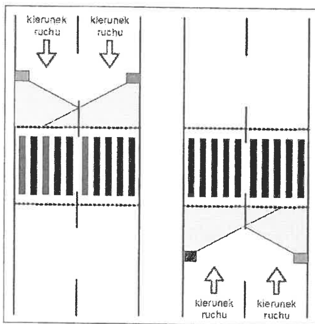
Rys. 2.2. Droga dwujezdniowa, układ prawo i lewostronny
